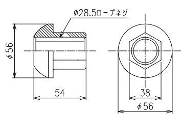
NNS突起付カプラ S=1/2
