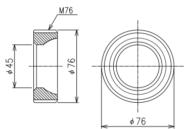
NNSキャップワッシャ S=1/2
