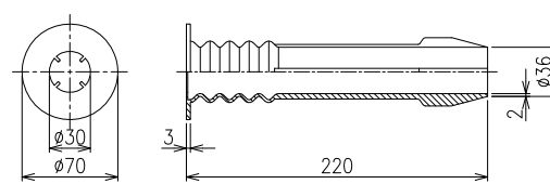
クランプW管 S=1/1
