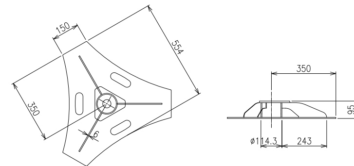
支圧板 S=1/10
