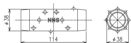
ファイヤロープ・ターンバックル S=1/3
