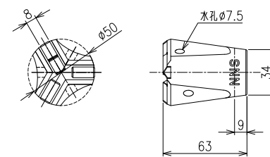
NNSビット S=1/2
