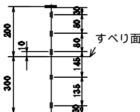
図2-2 補強材ひずみ計測位置
