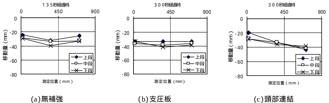
図3-3 地盤標点移動量
